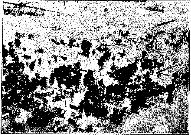
منظر مأخوذ من طائرة لمدينة « كوليس » في ولاية كنتكي في الولايات المتحدة وقد غمرتها مياه نهر المسيسيبي
